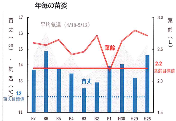
図 長岡普及指導センター調査7地点の平均値、品種はコシヒカリ、気温は長岡アメダス
